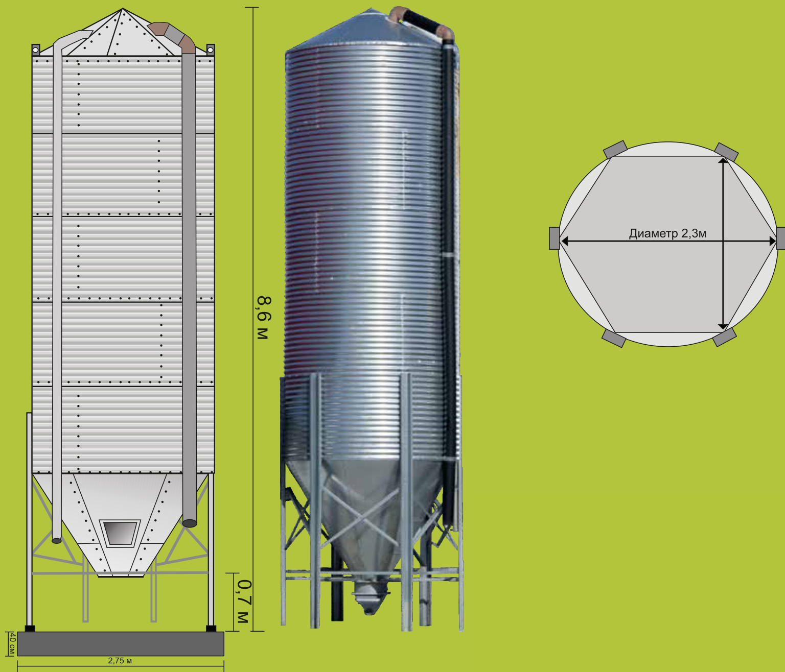
Бункеры SP-5
